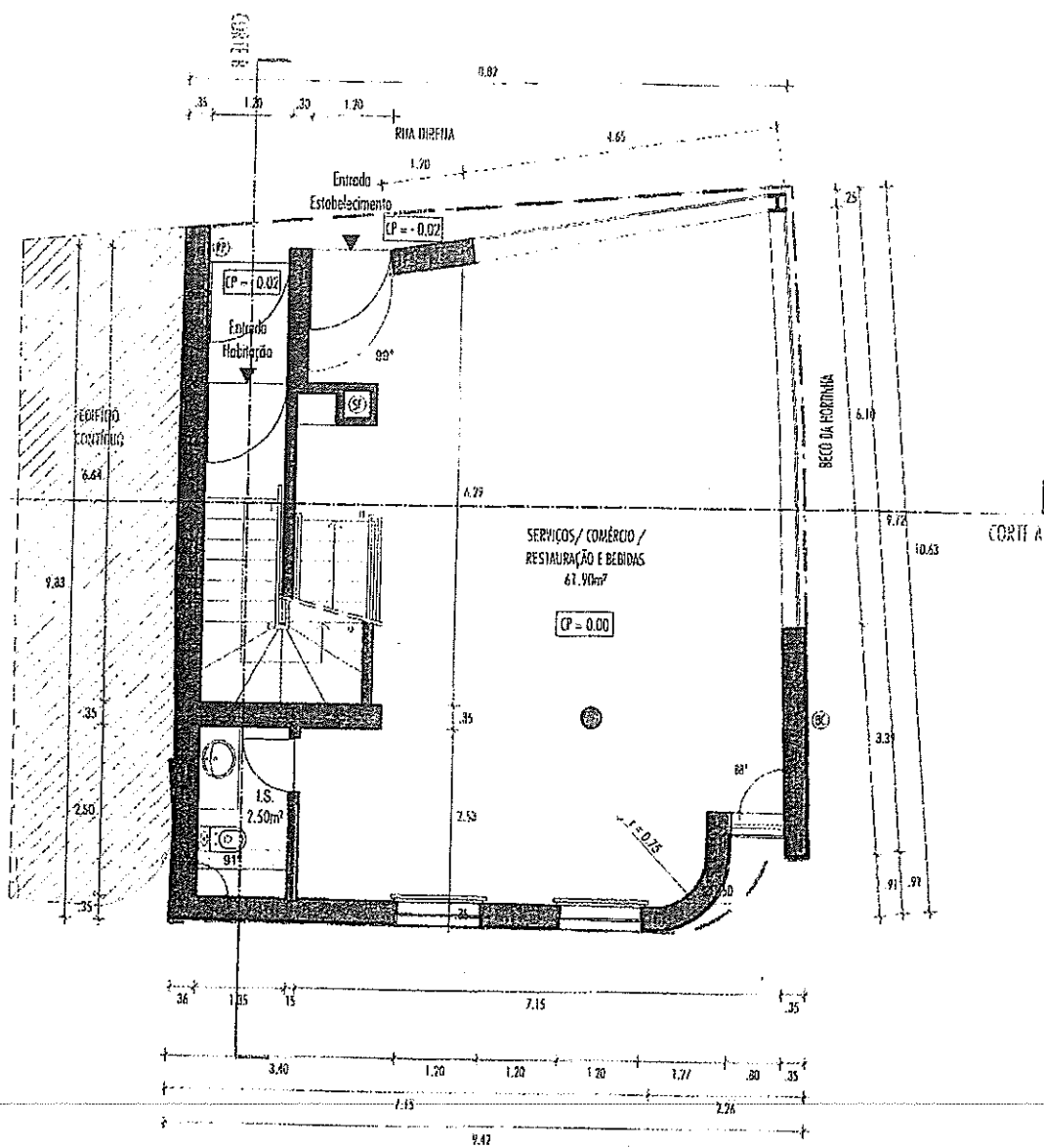
PLANTA DO R/C
