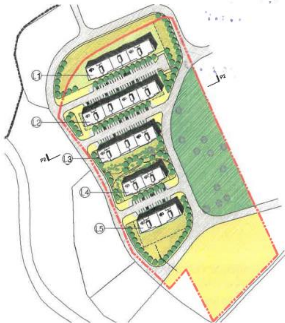
Fig. 2 – Planta sintese
