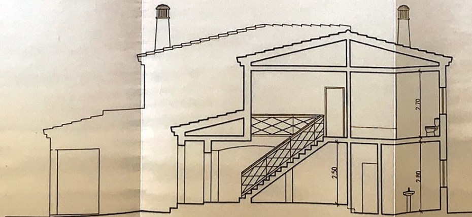
CORTE C-D
