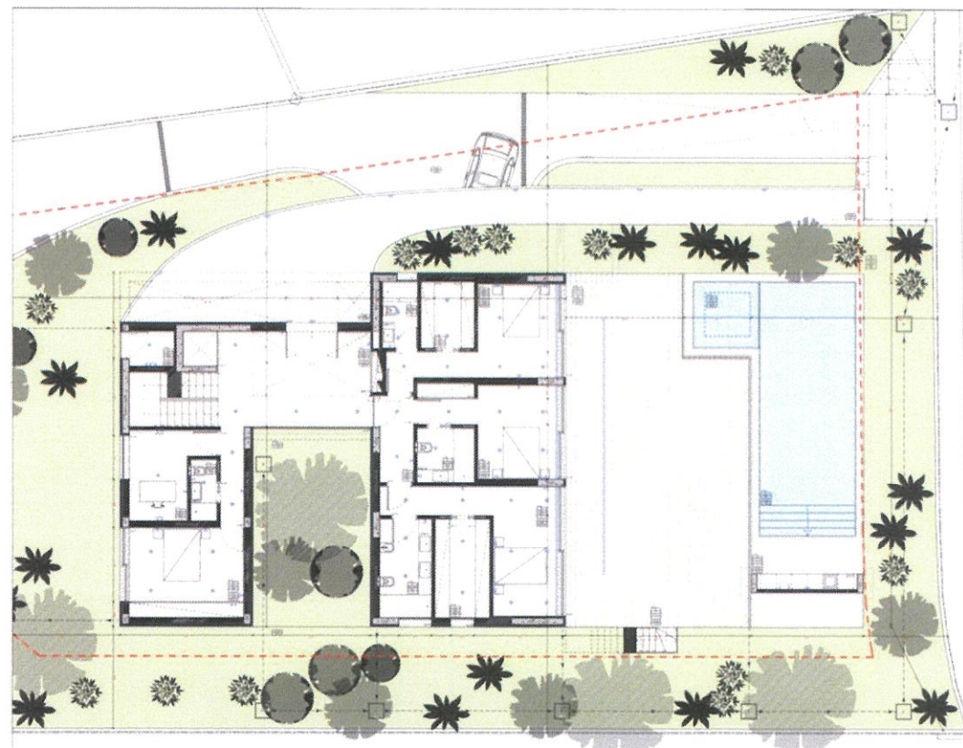
Rés-do-chão | 157m 2
