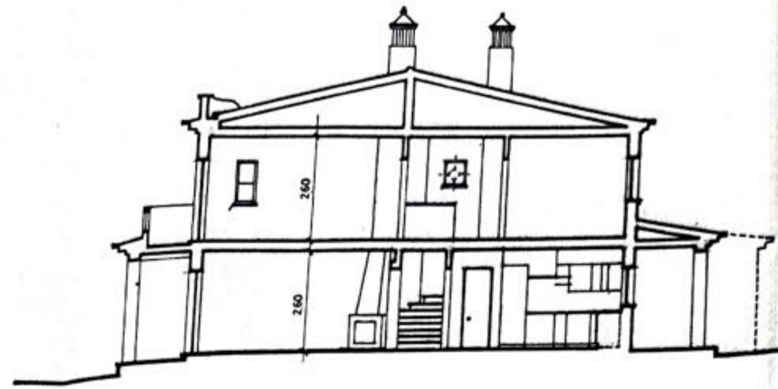
CORTE A-B
