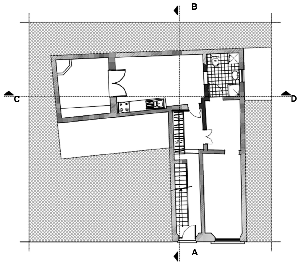
Planta do R/Chão
