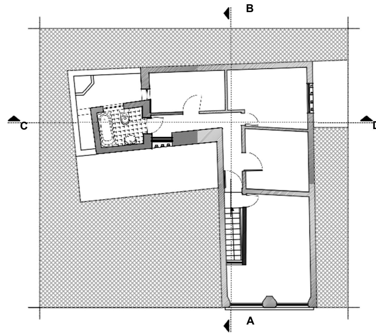
Planta do 1º Andar
