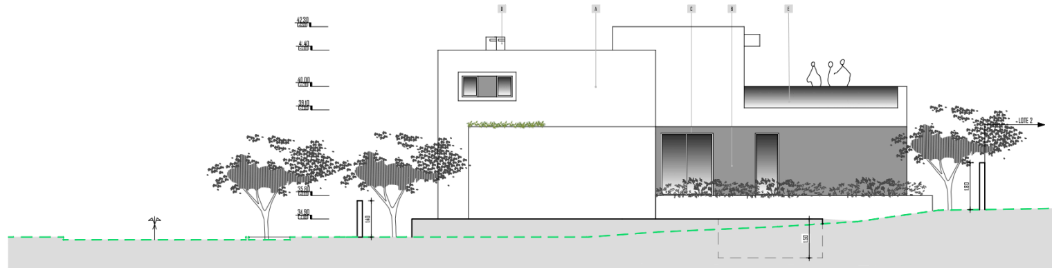
ALÇADO POSTERIOR
