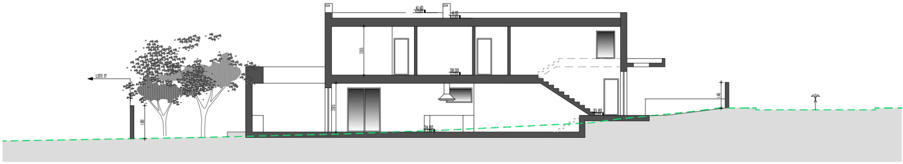
CORTE 1
