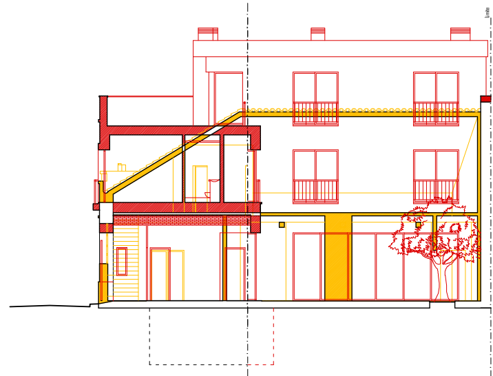
corte C2
