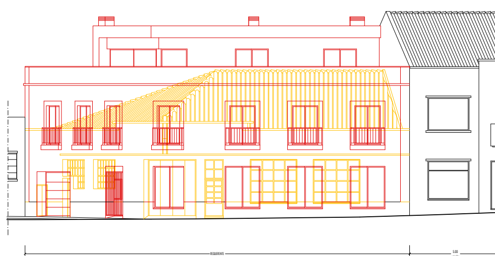
alçado A2
