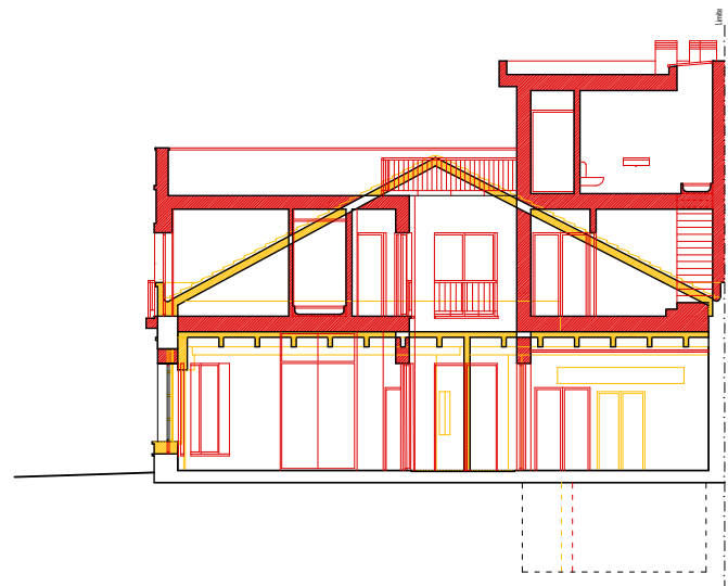
corte C1
