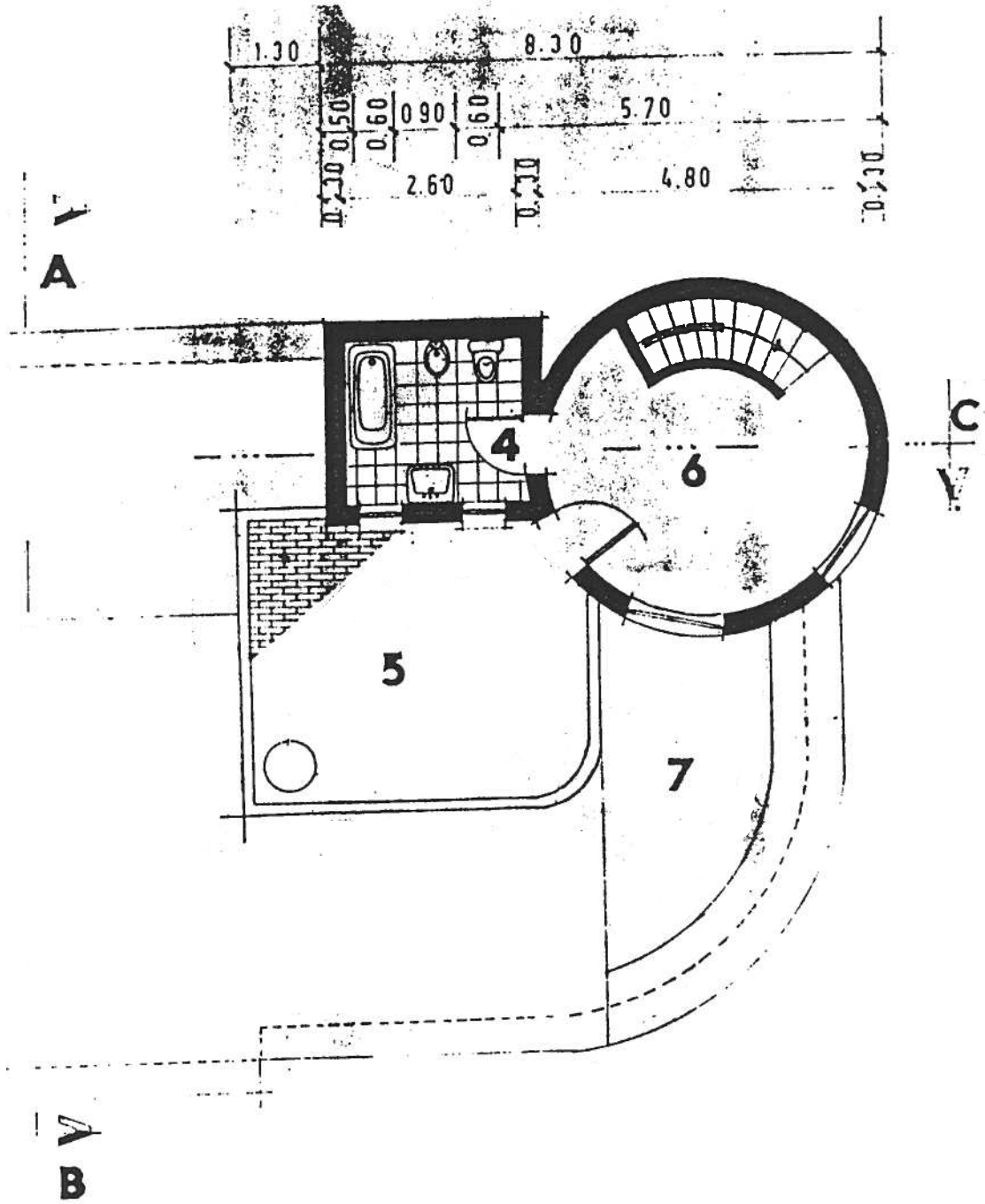
PLANTA • PISO SUPERIOR
