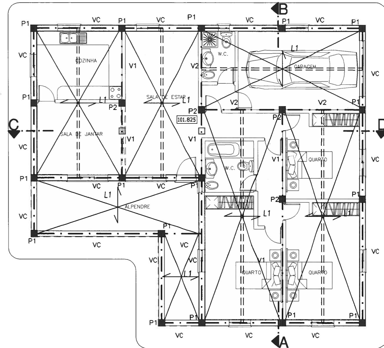
PLANTA DO PISO TÉRREO
