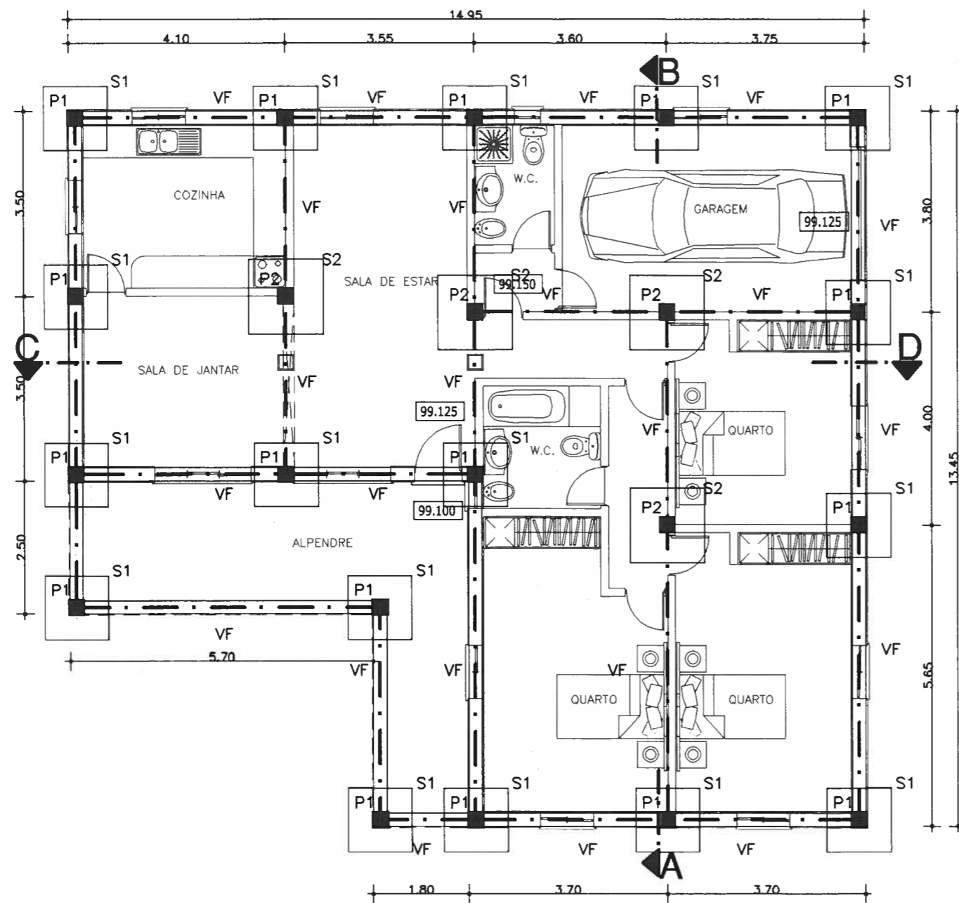
PLANTA DAS FUNDAÇÕES
