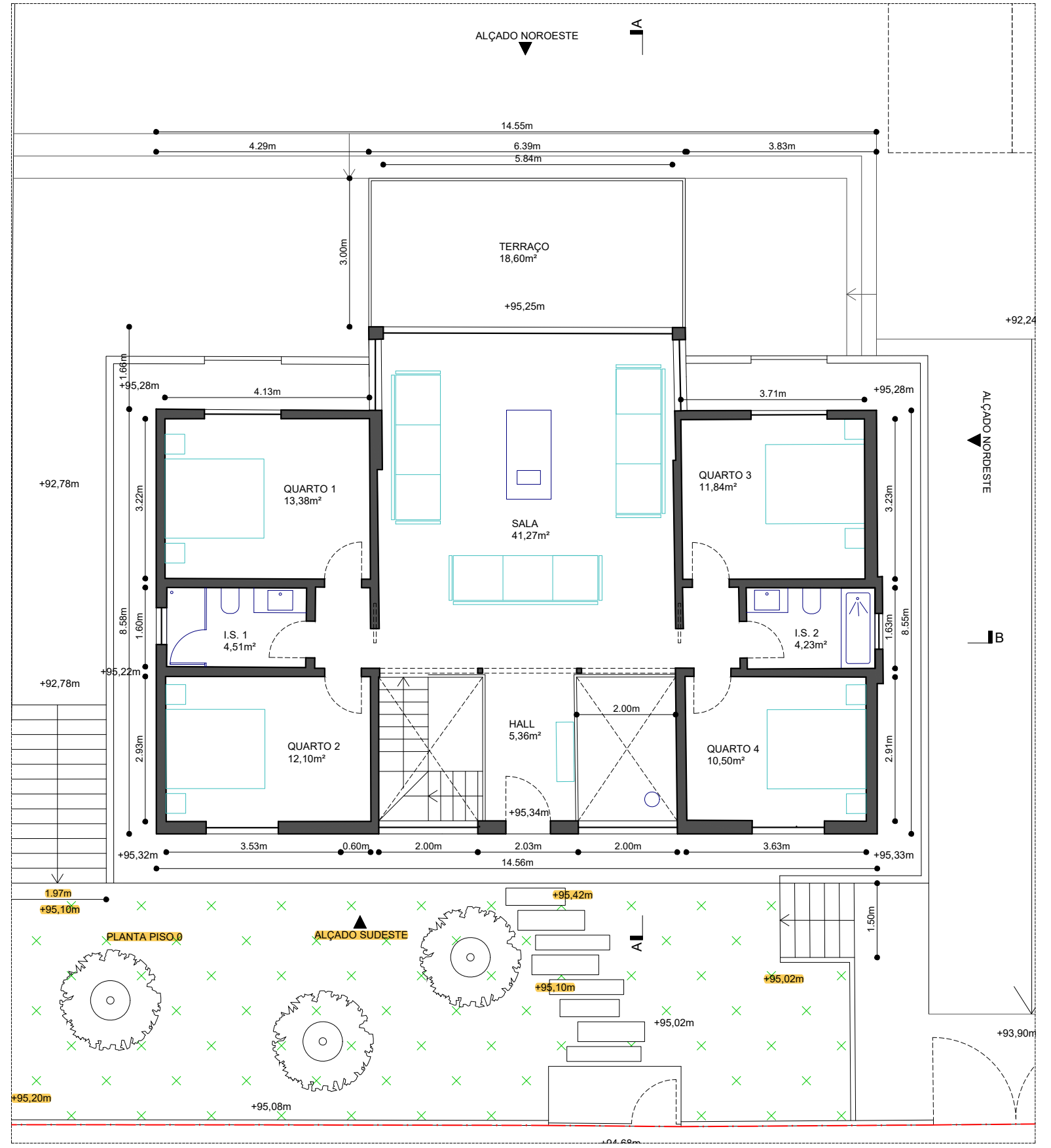
ESCALA 1:100
