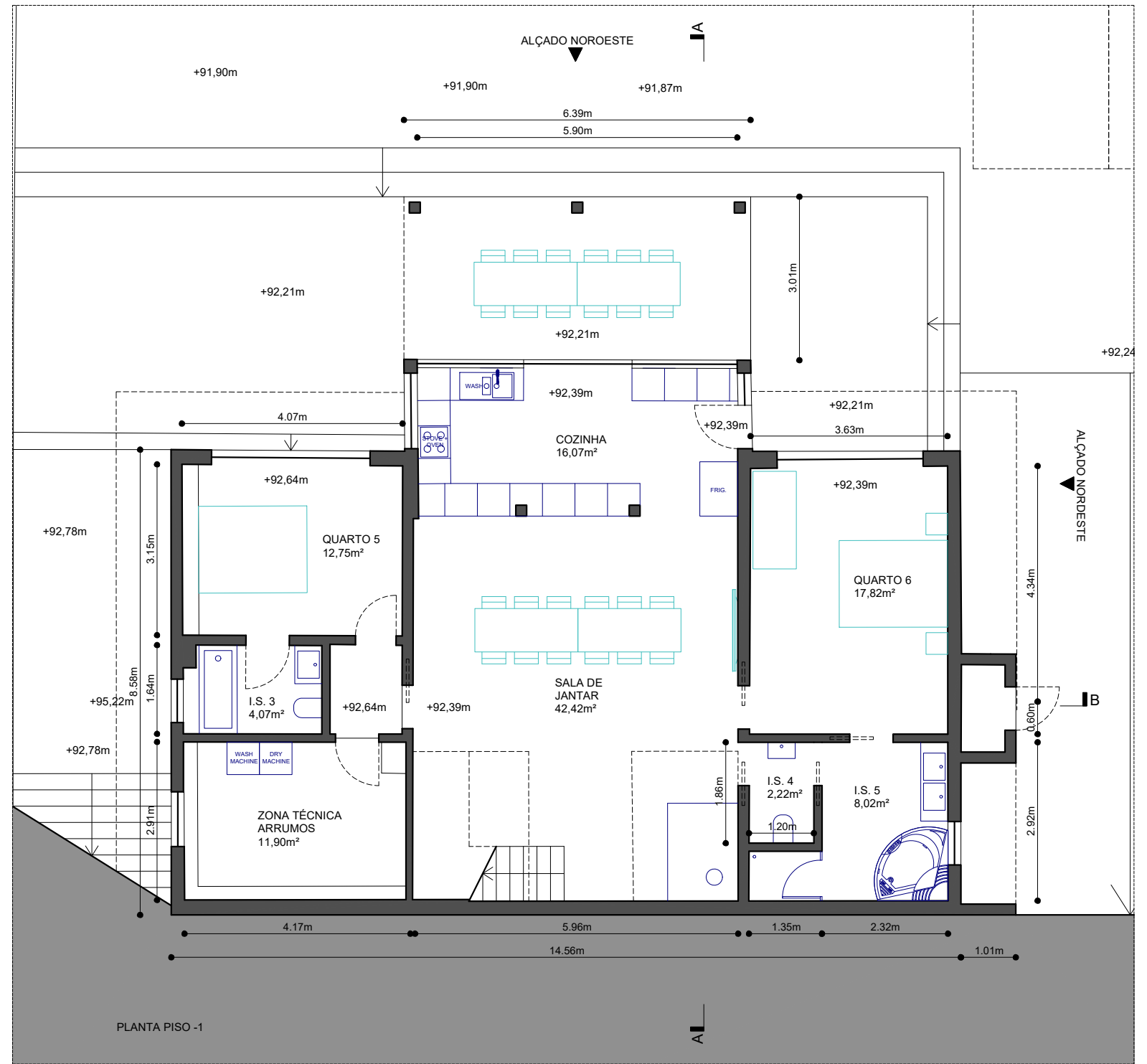
ESCALA 1:100
