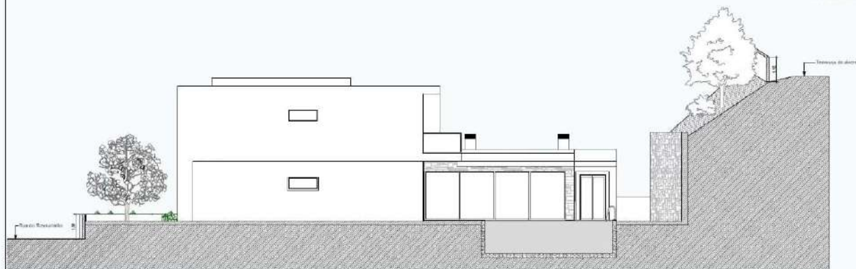
Poente Escala: 1:100
