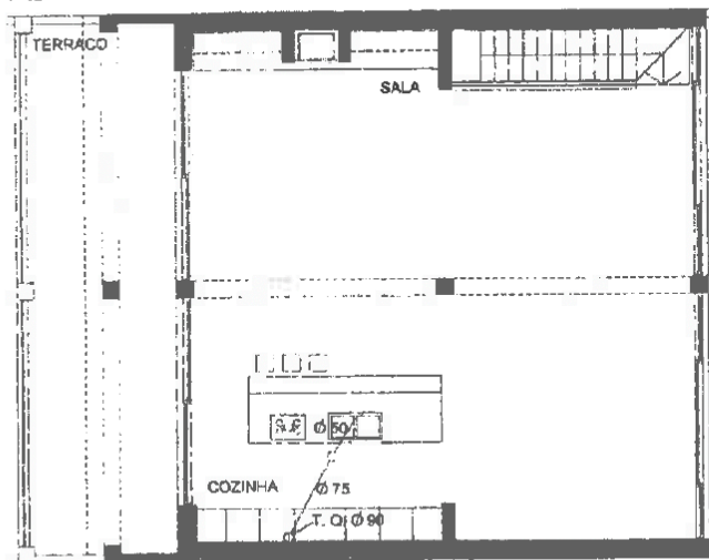
PLANTA DO R/CHÃO
