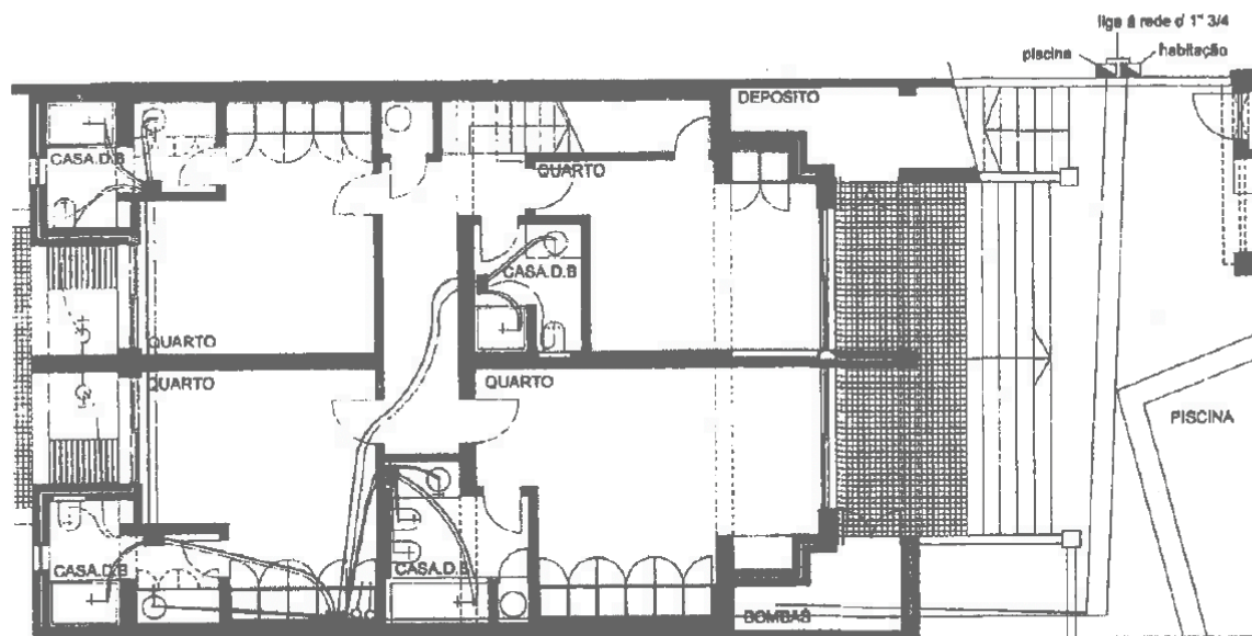
PLANTA DO R/CHÃO
