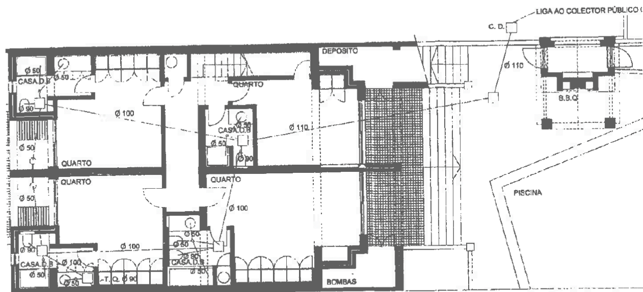
PLANTA DO R/CHÃO
